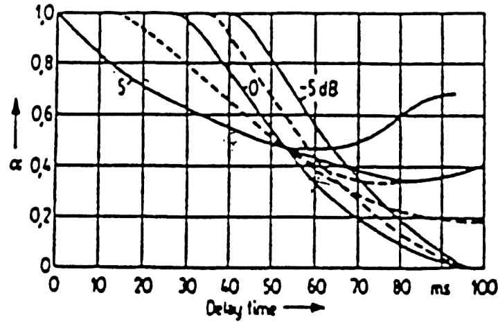
FIG. 2.8 - Fraction de l'énergie de la réflexion intégrée perçue à l'onde directe, en fonction du retard et paramétrée par le niveau de la réflexion.
