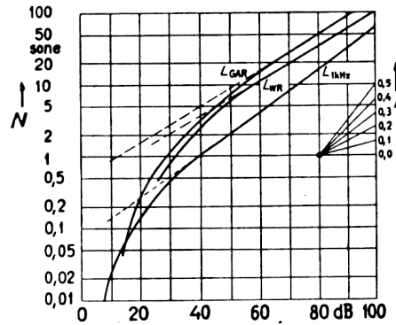
FIG. 2.5 - Sonie d'un son pur de 1 kHz, d'un bruit blanc et d'un bruit uniformément excitant, en fonction du niveau de pression acoustique, d'après [ZF81].
