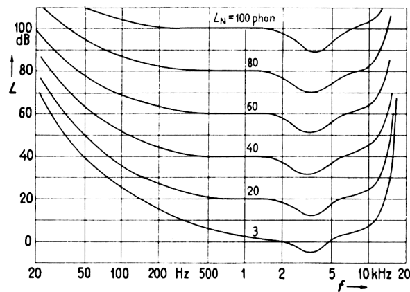
FIG. 2.9 - Courbes d'isophonie (en champs libre), d'après [ZF81].
