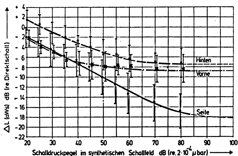
FIG. 2.6 - Seuil d'audibilité d'un écho (à 70 ms du son direct), en fonction du niveau sonore global, paramétré par la direction d'incidence : Vorne = incidence frontale, Hinten = incidence de l'arrière, Seite = incidence latérale.
