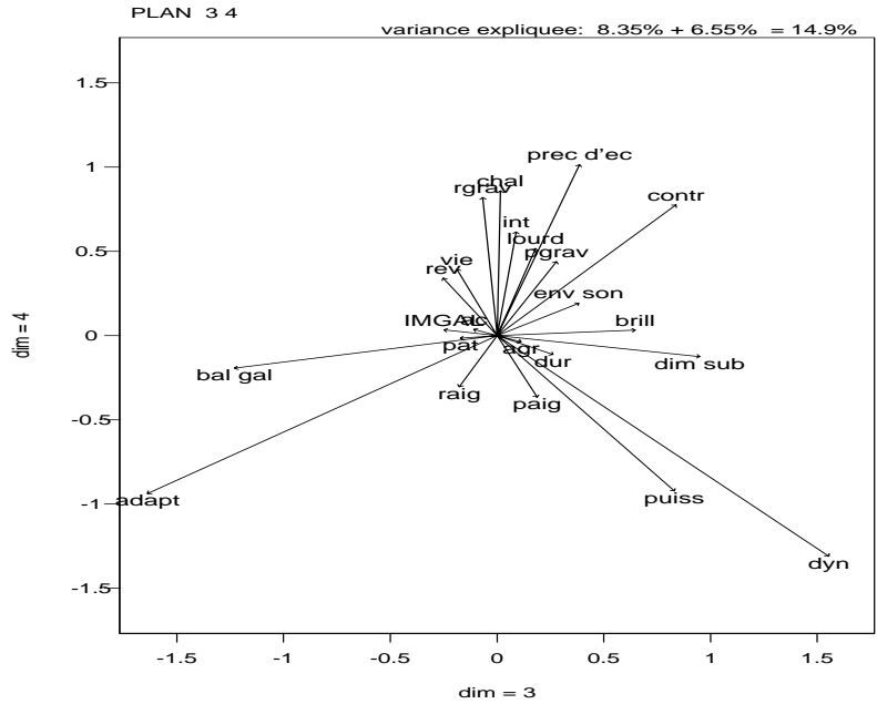
FIG. 6.12 - Plan 3/4 de l'ACP sur la somme des termes I(i_{m,k}) et R des réponses, itérées, aux questionnaires pour la campagne européenne des tests d'écoute. Les moyennes par place et par œuvre ont été enlevées.
