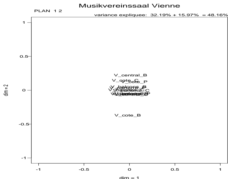
FIG. 6.18 - Musikvereinssaal Vienne : effet de l'interaction acoustique/œuvre. Les moyennes de sous-ensembles significatifs sont projetées dans l'ACP générale, figure 6.11. Les œuvres sont indiquées de la manière suivante : B pour l'oratorio de Noël de Bach, C pour le concerto pour piano et orchestre de Beethoven (avec couvercle enlevé) et P pour la symphonie Pastorale.
