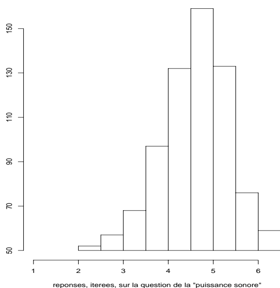
FIG. 5.1 - Histogramme des réponses sur la question de “puissance sonore”, pour la totalité de 383 jugements recueillis lors de la campagne européenne. On remarque surtout que le bas de l’échelle (le point 1 de l’échelle correspond à une puissance subjective très faible) n’est pas utilisé par les sujets, le centre de la distribution se trouve entre le point 4 (“assez forte”) et 5 (“forte”), et non pas au milieu de l’échelle, entre 3 (“assez faible”) et 4 (“assez forte”).
