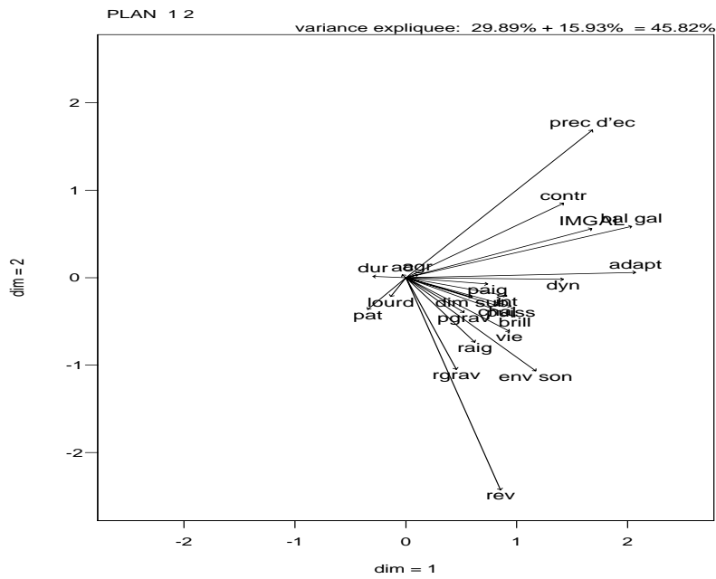
FIG. 6.11 - Plan 1/2 de l'ACP sur la somme des termes I(i_{m,k}) et R des réponses, itérées, aux questionnaires pour la campagne européenne des tests d'écoute. Les moyennes par place et par œuvre ont été enlevées.
