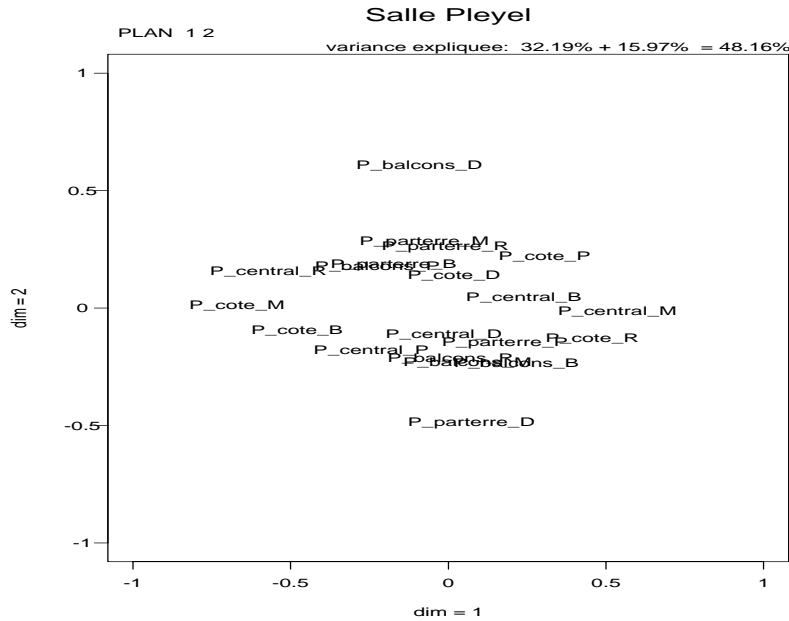
FIG. 6.17 - Salle Pleyel : effet de l'interaction acoustique/œuvre. Les moyennes de sous-ensembles significatifs sont projetées dans l'ACP générale, figure 6.11. Les œuvres sont indiquées de la manière suivante : M pour le concerto pour piano et orchestre de Mozart, B pour la symphonie de Beethoven, D pour la symphonie de Dutilleux, R pour l'ouverture de Rossini et P pour la musique de ballet de Prokofiev.
