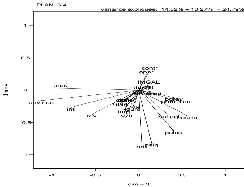
FIG. 5.3 - Plan 3/4 de l'ACP des réponses des sujets ayant appartenus au noyau stable de la campagne européenne de tests d'écoute, pour le premier test à la Villette, portant sur quatre répétitions de deux mouvements de la symphonie N° 39 de Mozart. Les moyennes des places étant enlevées, il s'agit uniquement du bruit restant contenu dans les réponses aux questionnaires, donc du terme \mathcal{R} .
